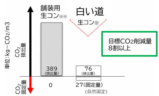
舗装材料1m3当たりCO2排出量試算***
